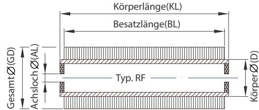
Typ Rundbürste mit eingesetztem Flansch
