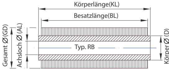
Typ Rundbürste Standard
