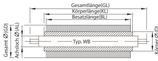
Typ Walzenbürste m. Welle Standard
