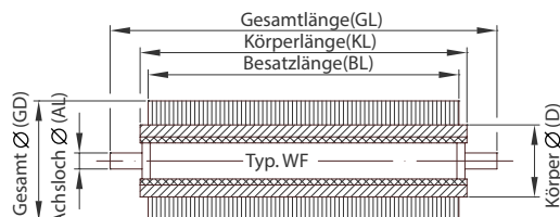
Typ Walzenbürste m. eingesetzten Achsenstummeln
